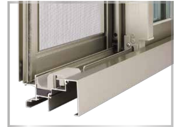
Sliding external insect screen บานมุ้งแบบติดตั้งด้านนอกห้องสำหรับบานเลื่อน
