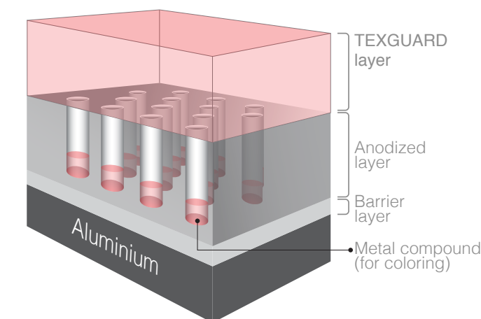
TOSTEM TEXGUARD ANODIZE
